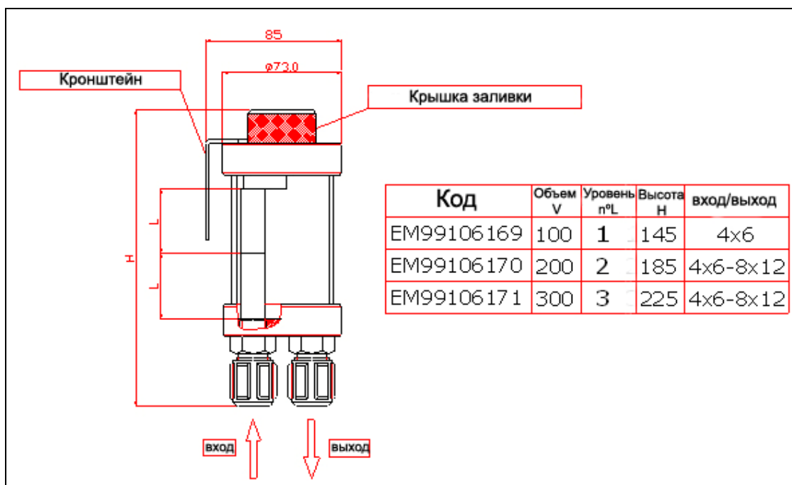
Рис. 1: Составные элементы и размеры
