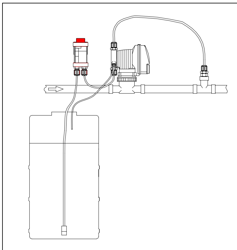
Рис. 2: Пример установки
