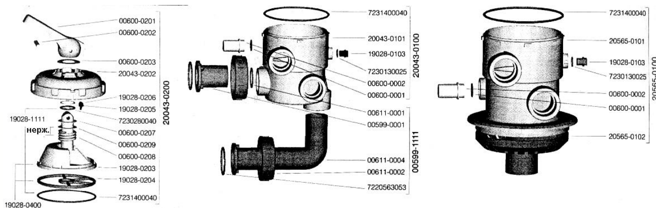
Многопозиционные вентили 1 1/2 дюйма
